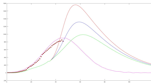
Figura 1. Cantidad de infectados en activo. Valor real \cdot , QLG, A.84, A.775, A.64.
